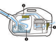
Triple filtrado: 1:filtro agua, 2:filtro intermedio lavable, 3:filtro HEPA 12
