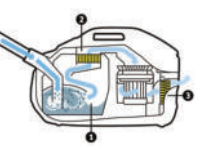
Triple filtrado: 1:filtro agua, 2:filtro intermedio lavable, 3:filtro HEPA 12
